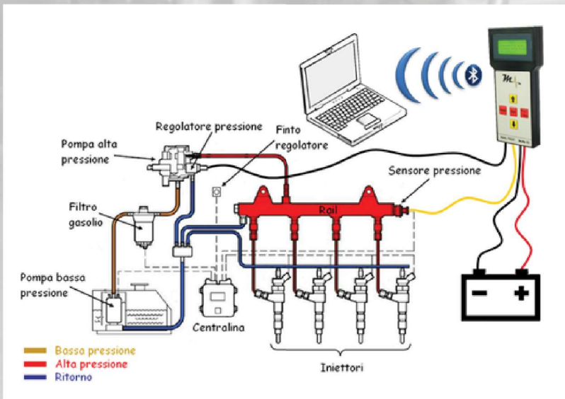
Collegamento MM03 su auto
