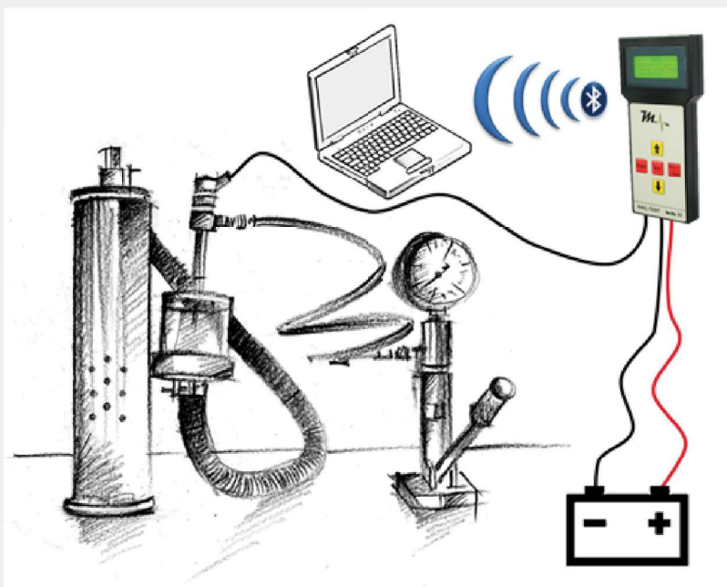
Collegamento MM03 al banco con aspiratore e pompa manuale
