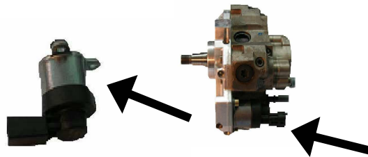
REGOLATORE FLUSSO BOSCH BOSCH FLOW REGULATOR
